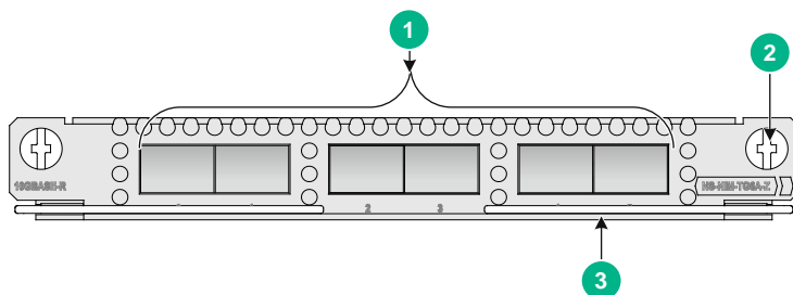
图A-7 NS-NIM-TG6A-Z 接口模块正视图
