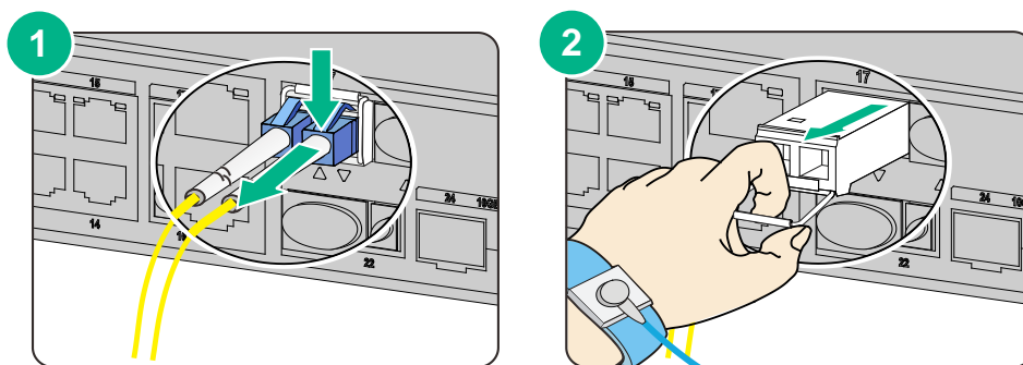
图4-5 拆卸光接口模块示意图
