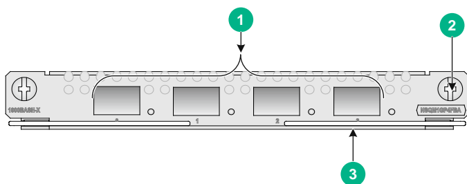
图A-6 NSQM1GP4FBA 接口模块正视图
