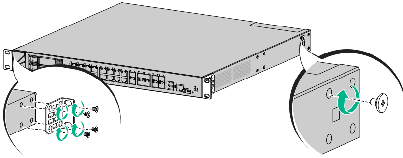
图2-4 安装前挂耳和承重螺钉
