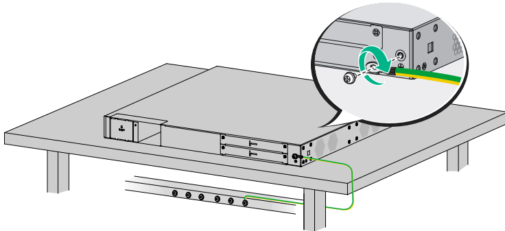
图2-6 通过接地排接地
