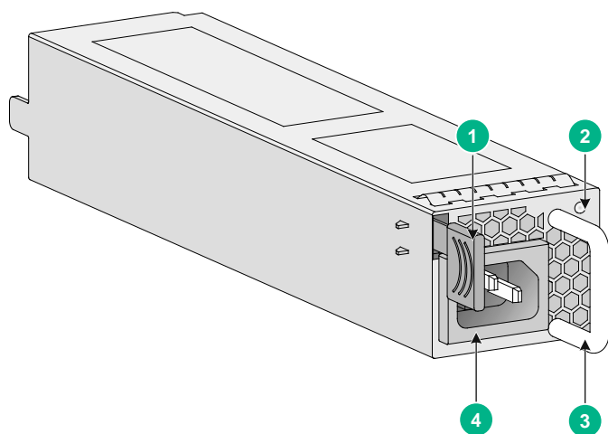
图A-8 PSR250-12A1-Z 交流电源模块外观
