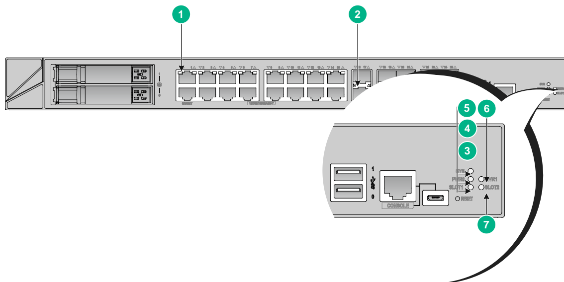
图B-1 F1000-CN80 指示灯
