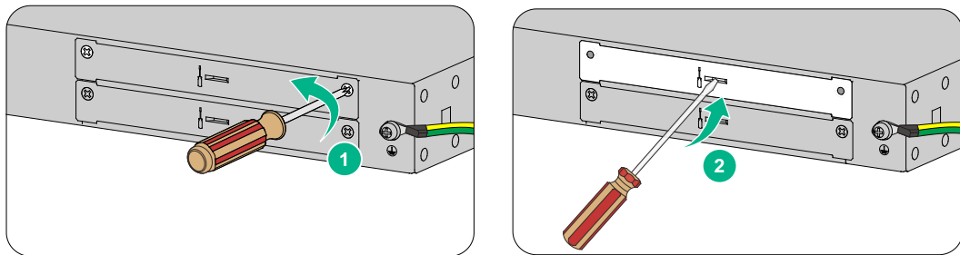
图2-10 拆卸假面板
