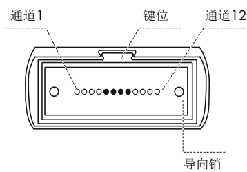
图1-2 12 芯光纤的 MPO 连接器俯视图
