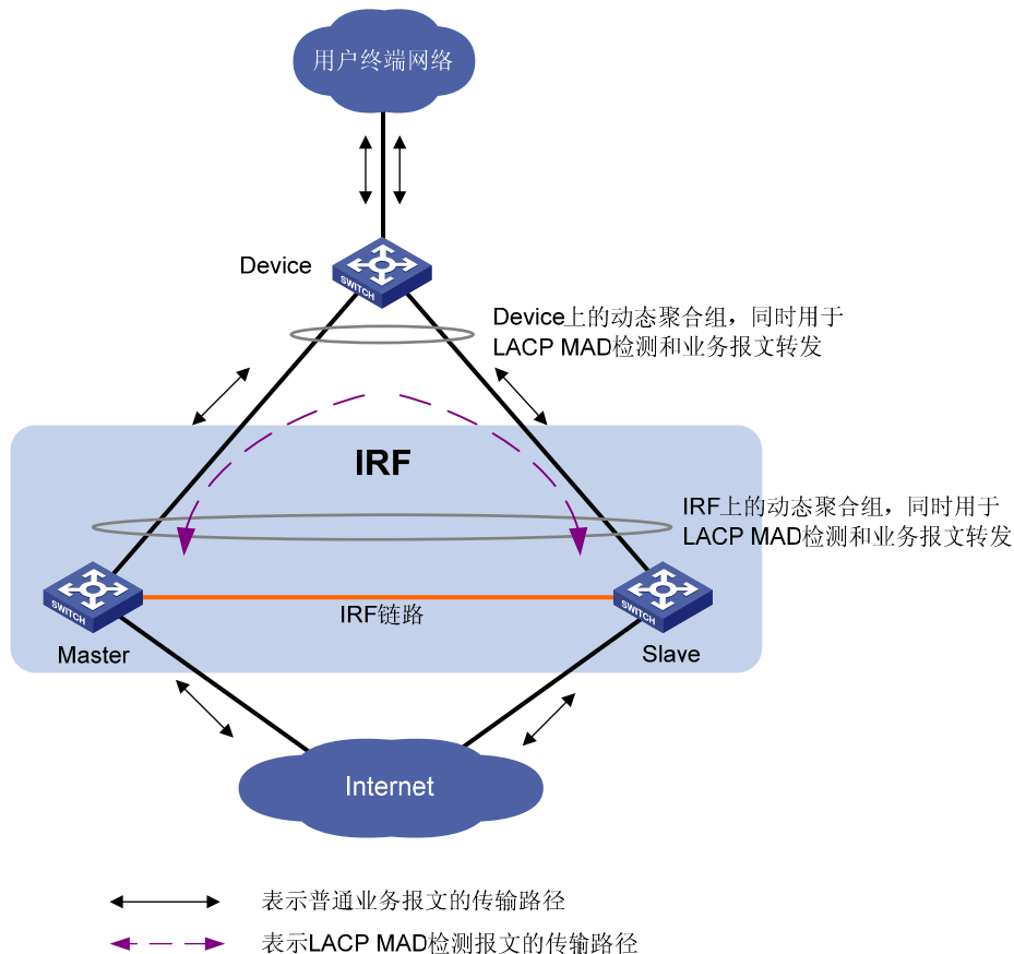
图1-8 LACP MAD 检测组网示意图
