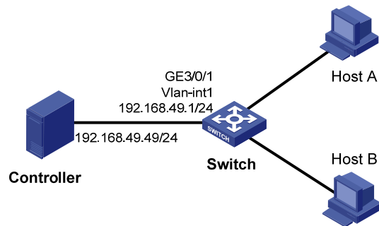
图1-7 OpenFlow 配置组网图
