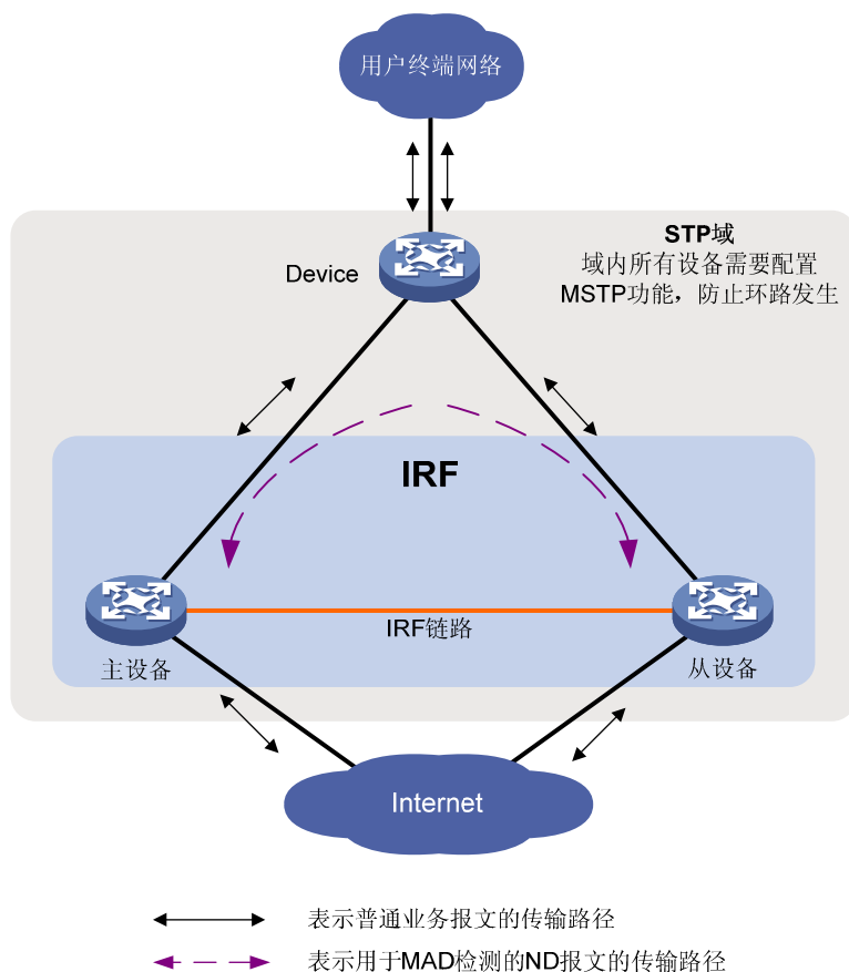
图1-10 ND MAD 检测组网示意图
