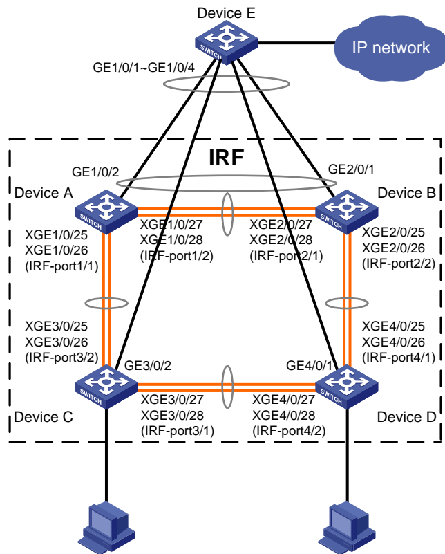
图1-13 IRF 典型配置组网图（LACP MAD 检测方式）
