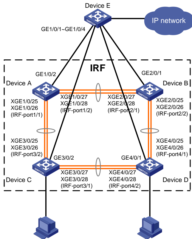
图1-15 IRF 典型配置组网图（ARP MAD 检测方式）
