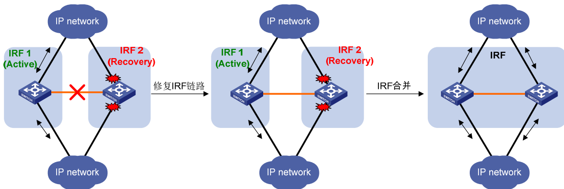
图1-11 MAD 故障恢复（IRF 链路故障）
