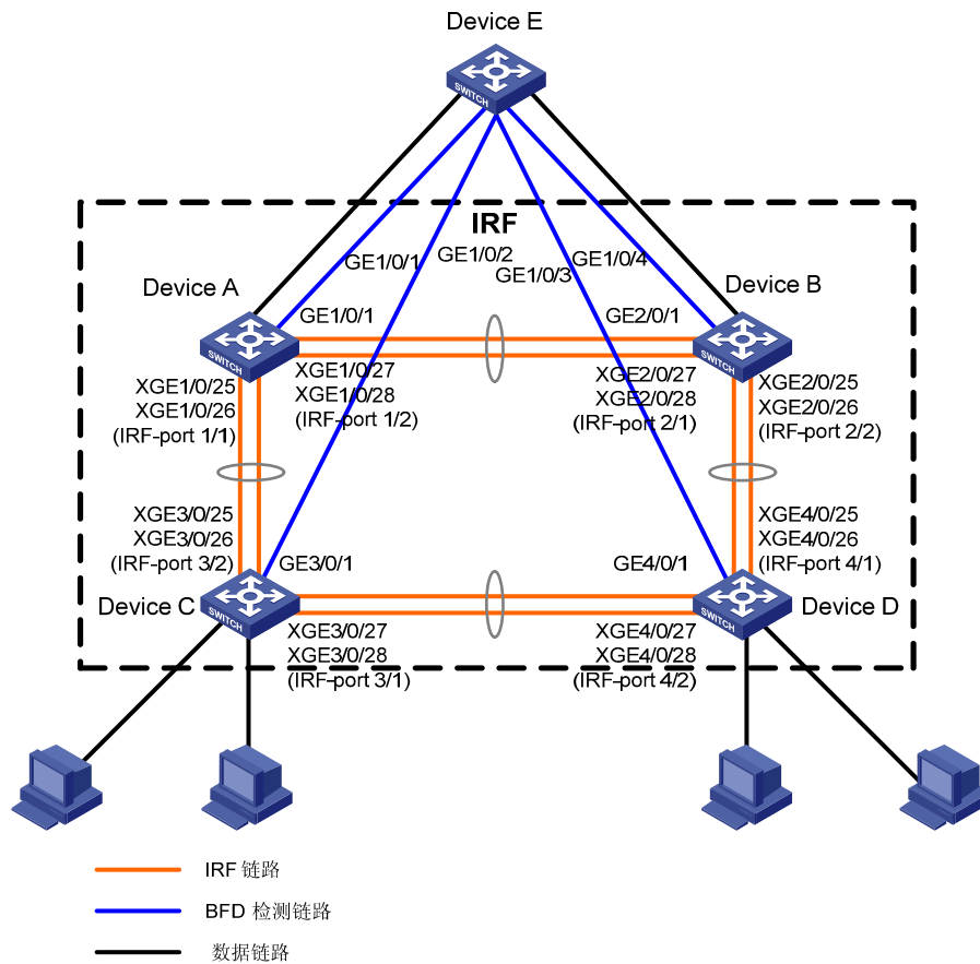
图1-14 IRF 典型配置组网图（BFD MAD 检测方式）
