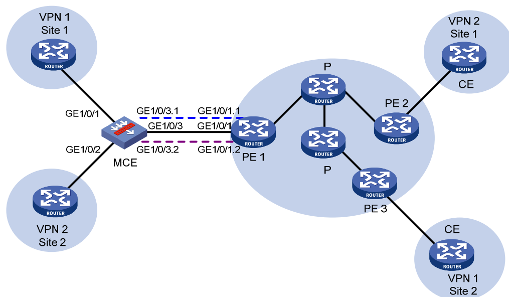
图1-3 MCE 工作原理示意图
