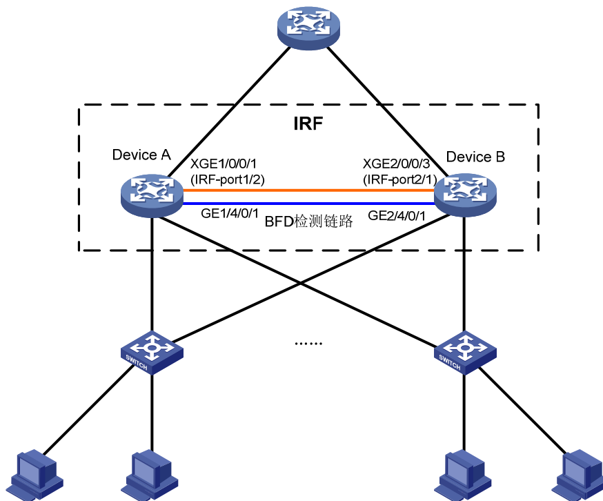
图1-13 组建 IRF 典型配置组网图（BFD MAD 检测方式）
