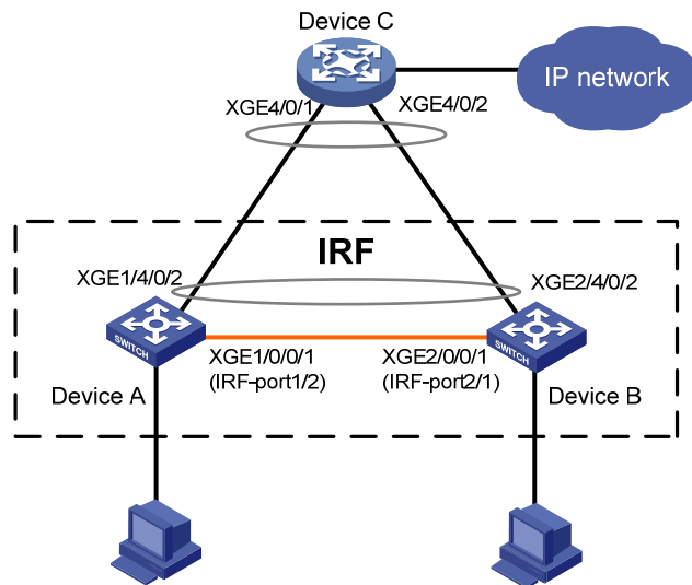
图1-12 组建 IRF 典型配置组网图（LACP MAD 检测方式）
