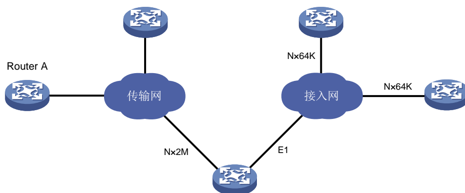
图1-1 CPOS E1/T1/E3/T3 接口典型应用组网图
