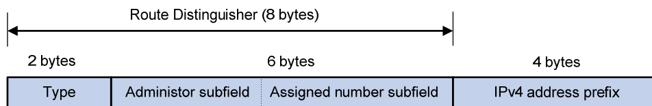
图1-2 VPN-IPv4 地址结构
